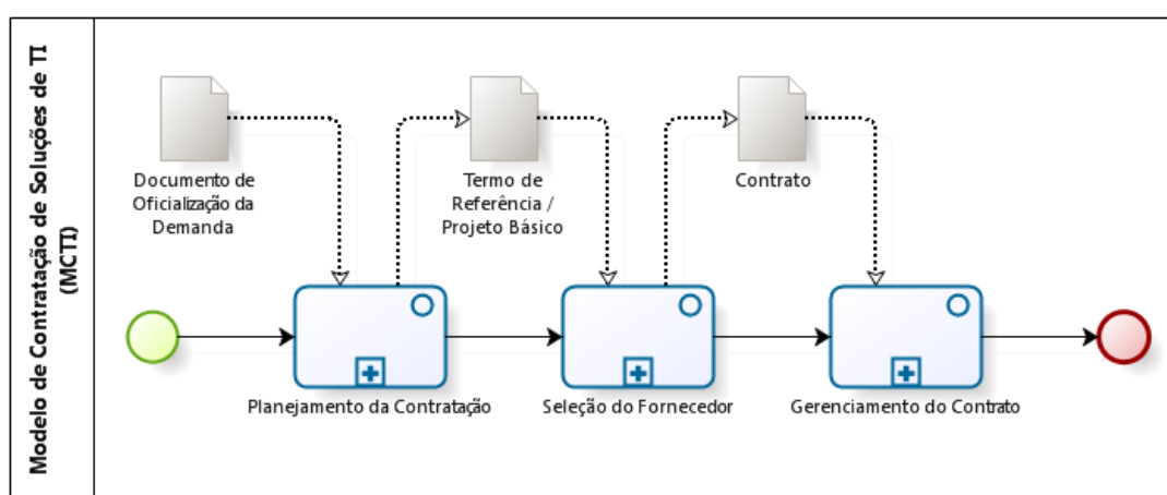
Figura 2: Modelo de Contratação de Soluções de TI
